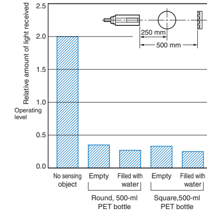
E3F□-B□1
