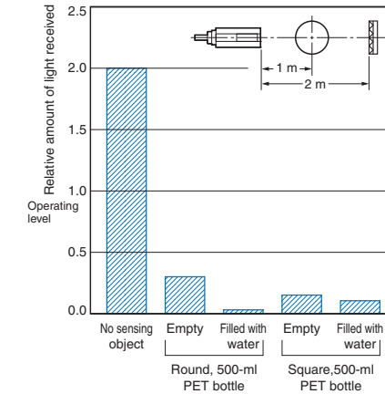
E3F□-B□2
