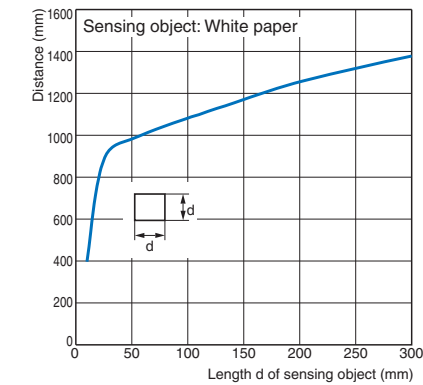
E3FA-D□6
