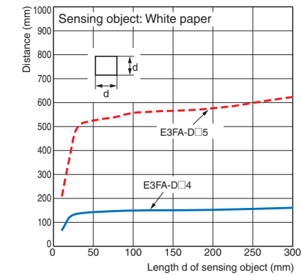
E3FA-D□4, E3FA-D□5
