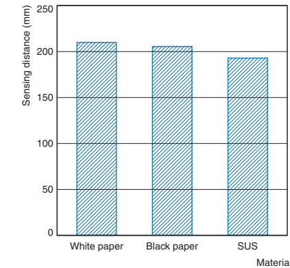
E3F□-L□2
